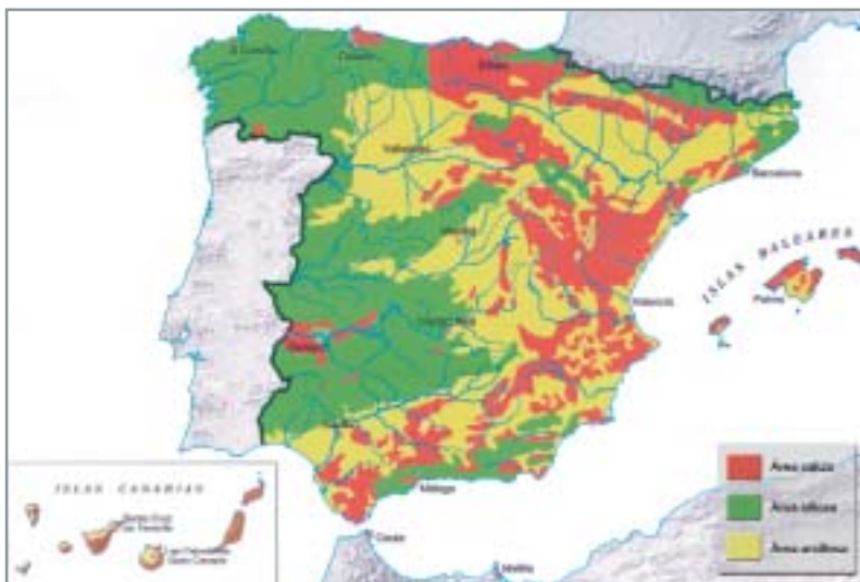
El roquedo peninsular.
