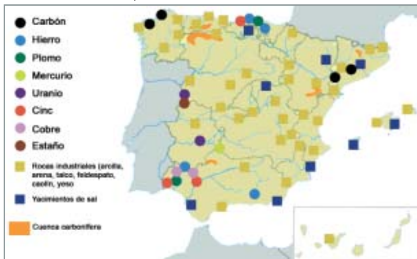
Recursos minerales en España
